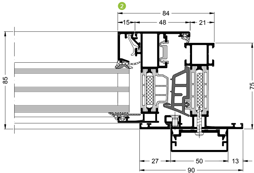
Blendrahmen Flügel aufschlagend Outer frame with face-fitted vent
