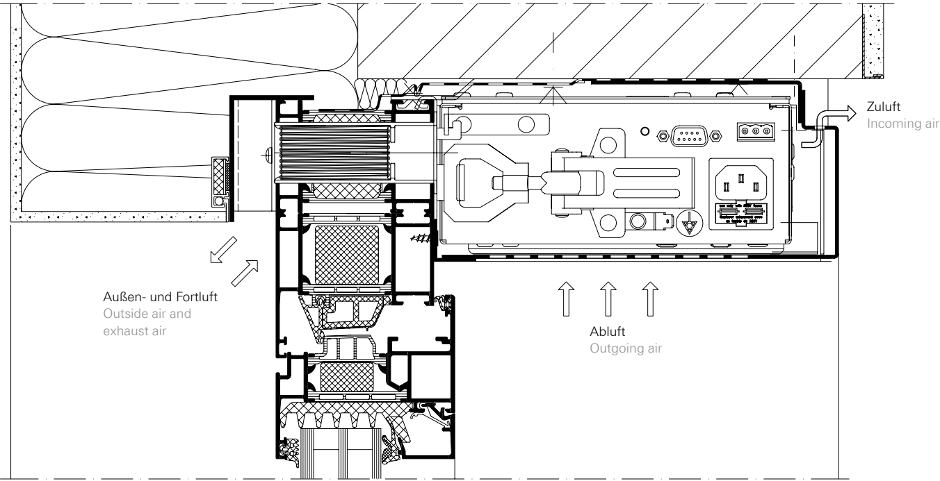
Schüco VentoTherm in Schüco AWS 75.SI+ Schüco VentoTherm in Schüco AWS 75.SI+
