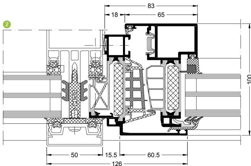
Einsatzblendrahmen für Fassaden Insert outer frame for façades
