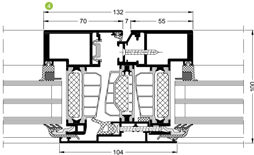
Stulp Double vent
