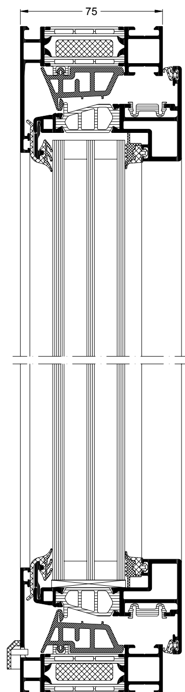
Schüco Fenster AWS 75 BS.HI+ Schüco Window AWS 75 BS.HI+
