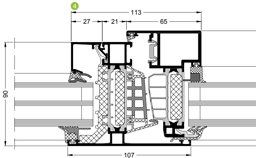
Flügel mit Festfeld Vent with fixed light
