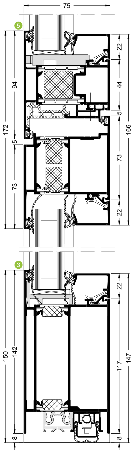
Tür mit oberem Festfeld, flächenbündig, 1-flügelig, nach innen öffnend Door with fixed light at top, flush-fitted, single-leaf, inward-opening
