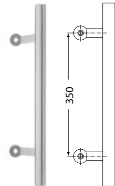
Türgriff gerade Straight door pull
