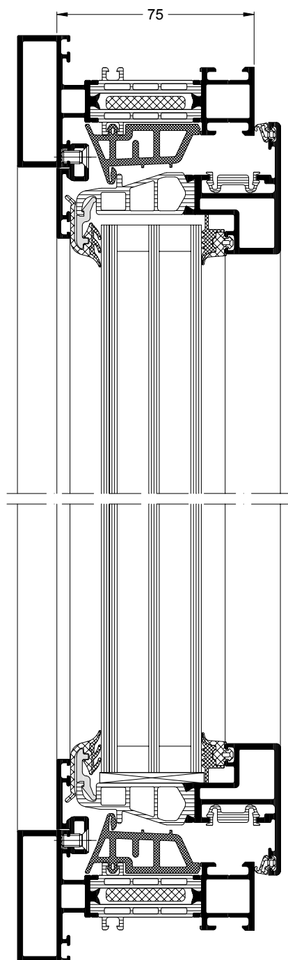
Schüco Fenster AWS 75 WF.SI+ Schüco Window AWS 75 WF.SI+
