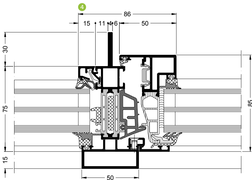
Statikpfosten Flügel aufschlagend Structural mullion with face-fitted vent
