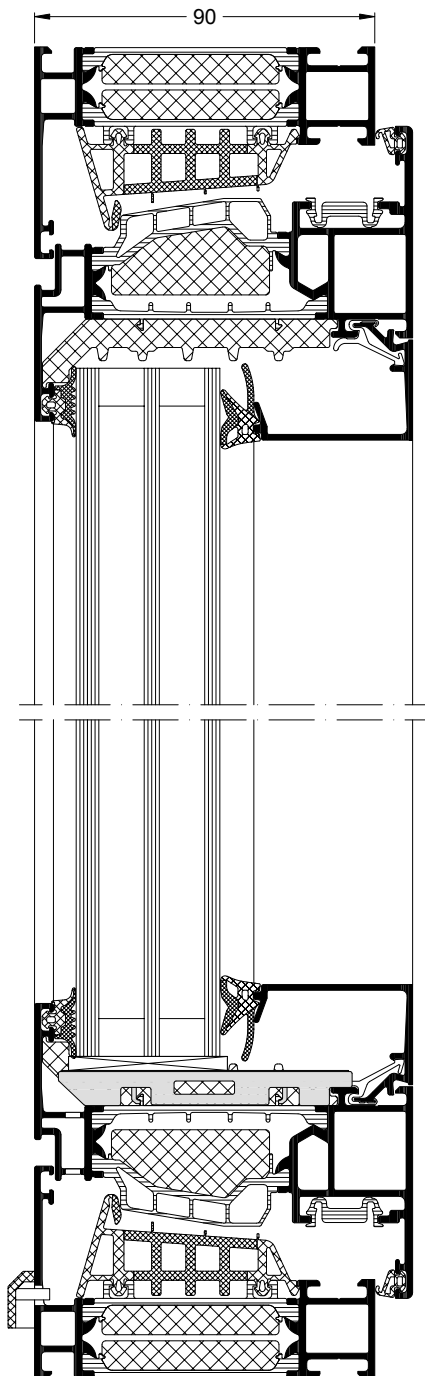
Schüco Fenster AWS 90.SI+ / AWS 90.SI+ Green Schüco Window AWS 90.SI+ / AWS 90.SI+ Green
