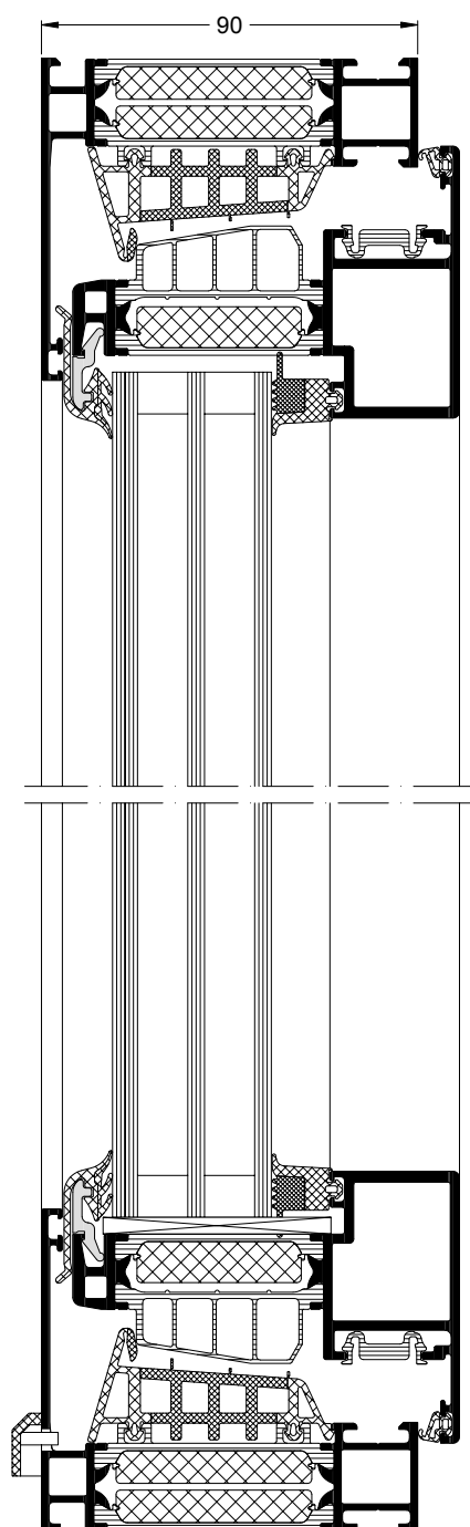
Schüco Fenster AWS 90 BS.SI+ Schüco Window AWS 90 BS.SI+
