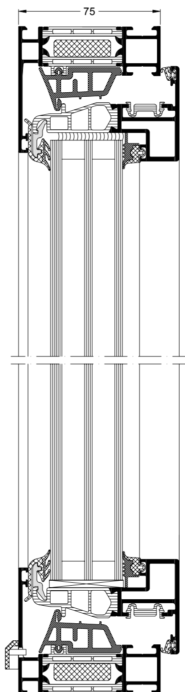
Schüco Fenster AWS 75 BS.SI+ Schüco Window AWS 75 BS.SI+
