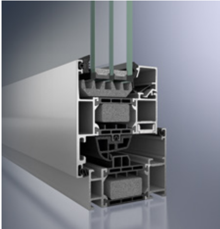
Schüco Fenster AWS 75.SI+, außen öffnend Hochisoliertes Fenstersystem als neuer Wärme- dämmstandard unter den außen öffnenden Fensterreihen.
